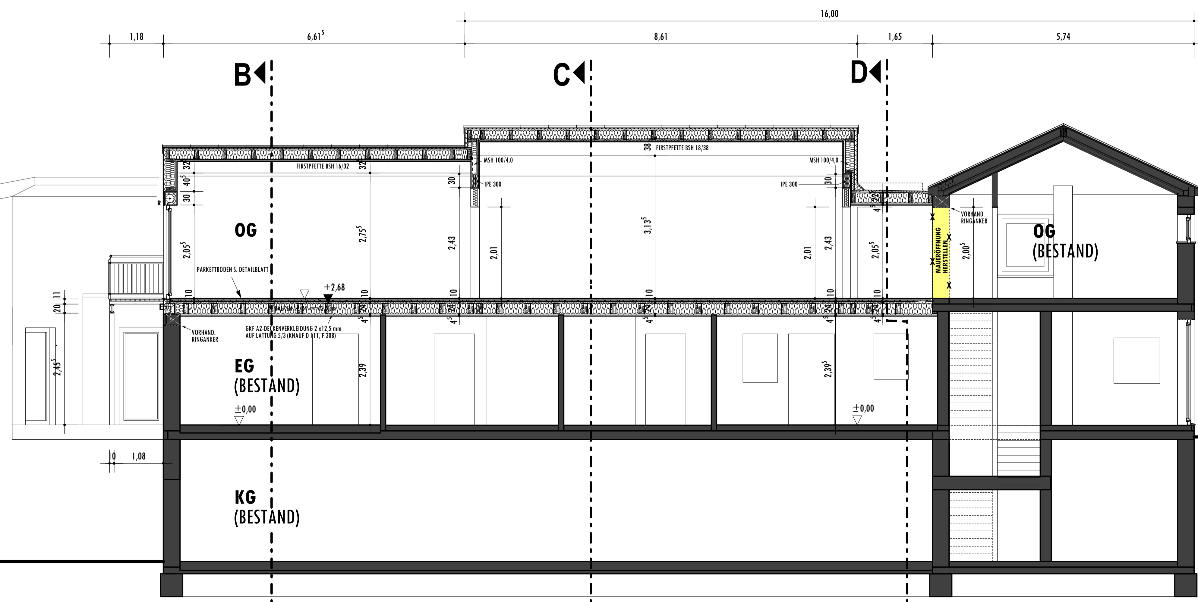
SCHNITT A-A
